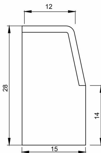
Bordillo Calzada C4
