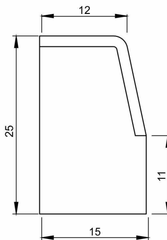
Bordillo Calzada C5
